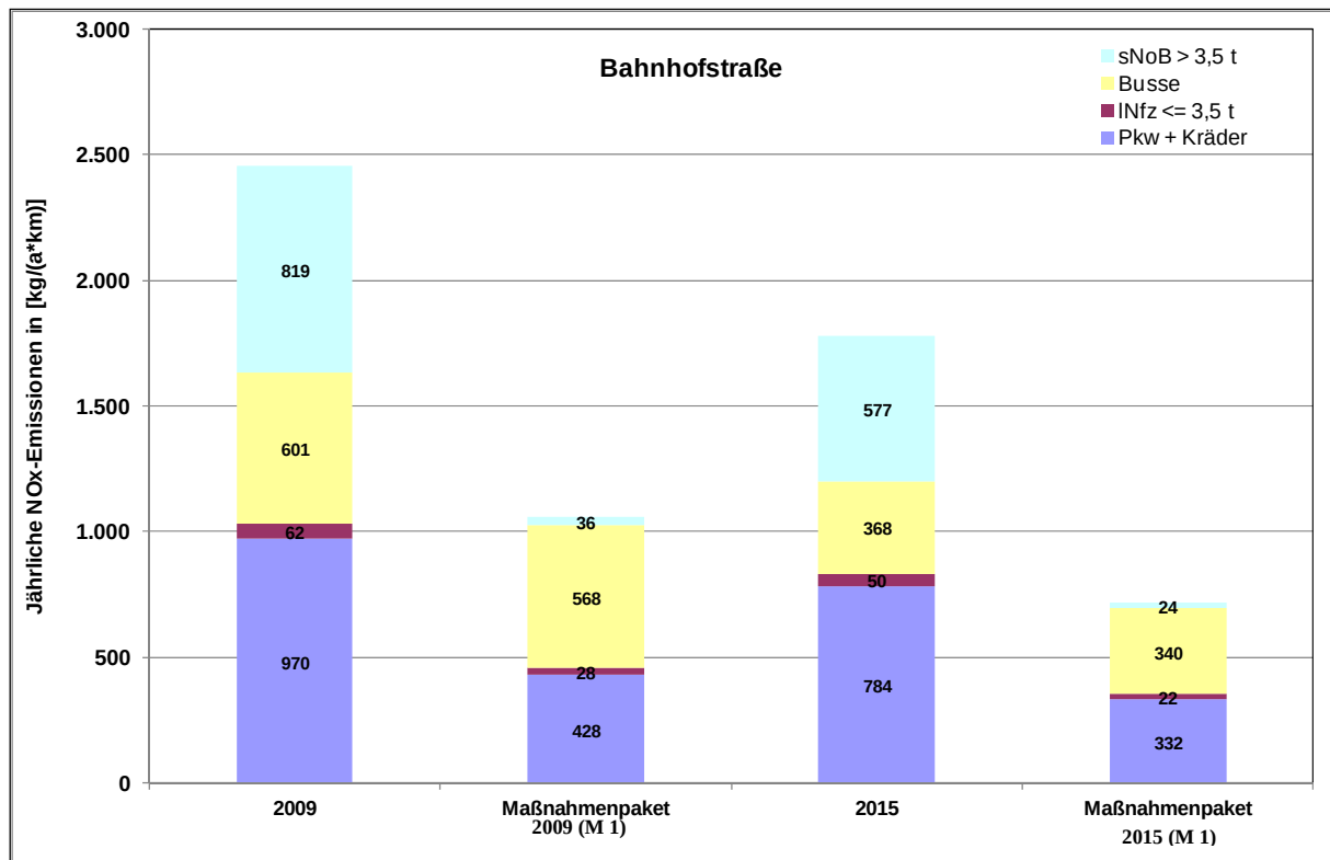
(28) Abb. 6.2/1: NO x -Emissionsanteile verschiedener Fahrzeugarten für die Bahnhofstraße (Analyse 2009, Trend 2015 u. Maßnahmenpaket (M 1))
