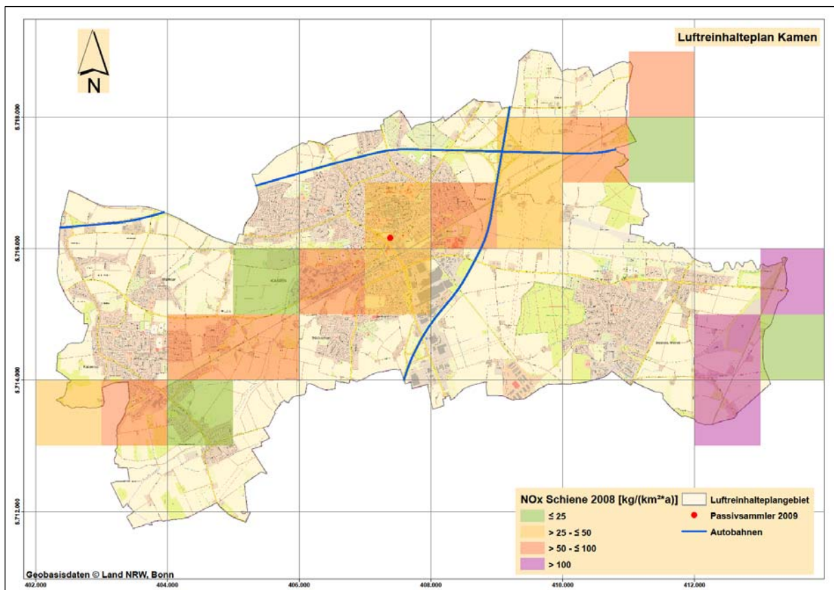
(12) Abb. 3.2.2/3: NO x -Emissionen des Schienenverkehrs im LRP-Gebiet (Datenbasis 2008)
