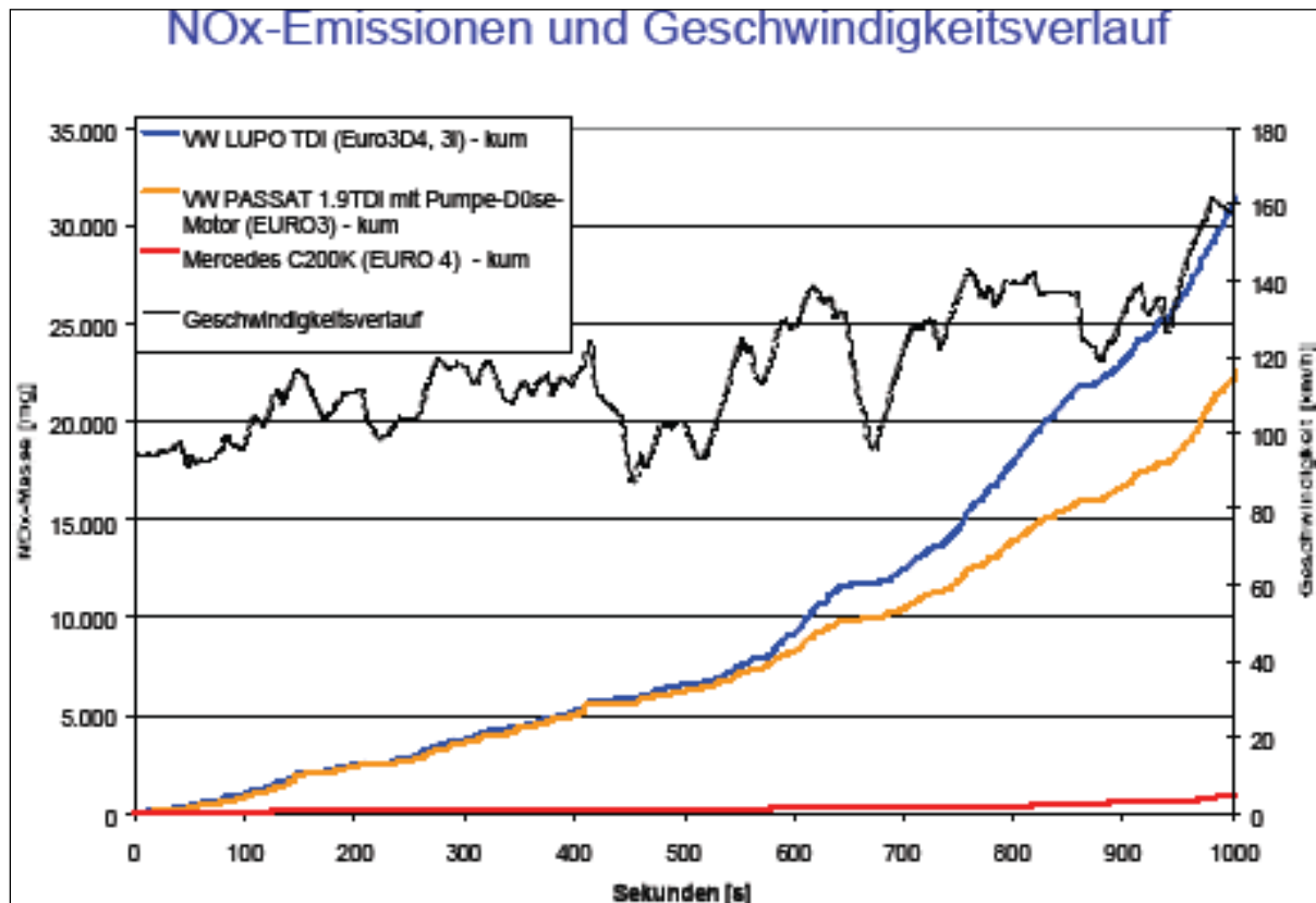
(30) Abb. 7.1/1: kumulierte \text{NO}_x -Emissionen von zwei Diesel-Pkw im Vergleich mit einem Otto-Pkw in einem Autobahnzyklus, der bis 160 km/h reicht 51
