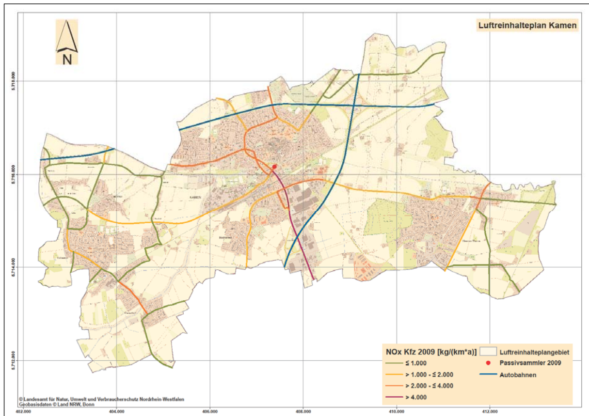
(10) Abb. 3.2.2/2: NO x -Emissionen des Kfz-Verkehrs im LRP-Gebiet (Datenbasis 2009)
