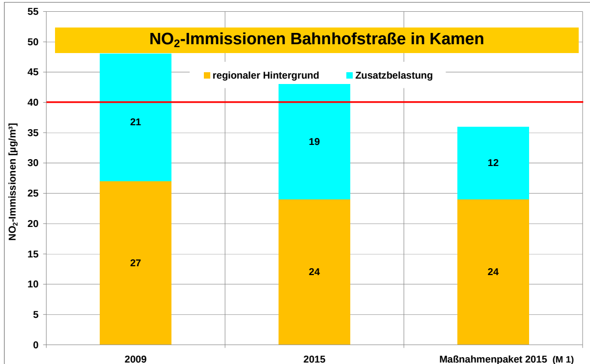
(29) Abb. 6.3/1: NO 2 -Immissionsprognose für die Bahnhofstraße 2009 & 2015 (o. & mit Maßnahmen)
