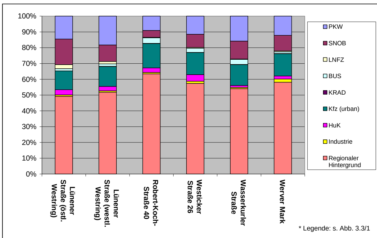
(18) Abb. 3.3/2: Prozentual berechnete Beiträge (2009) der verschiedenen Verursacherguppen sowie des regionalen Hintergrunds für die NO x -Belastung an einer repräsentativen Auswahl an Straßen aus den Verdachtsfällen der Stadt Kamen
