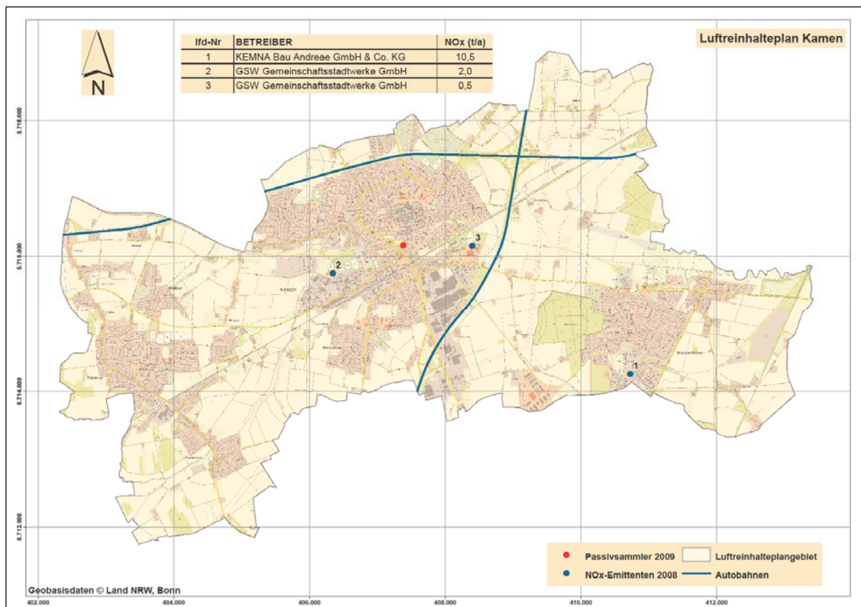
(14) Abb. 3.2.3/1: NO x -Emissionen der nach dem BImSchG genehmigungsbedürftigen Anlagen der Industrie im LRP-Gebiet
